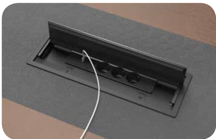
Инто Про — лючок для вывода проводов с двусторонним открыванием в комплекте с розеточным блоком: 3 силовые розетки + USB (A+C) + Cat6 + HDMI, кабель питания 1,8 м
